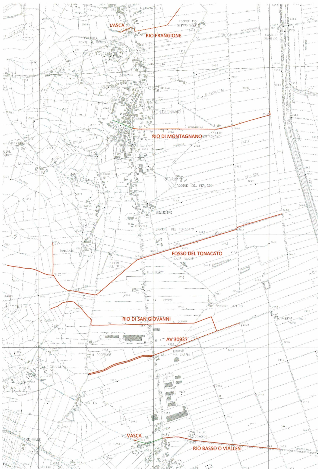
Figura 1 - Planimetria con indicazione dei tratti di intervento
